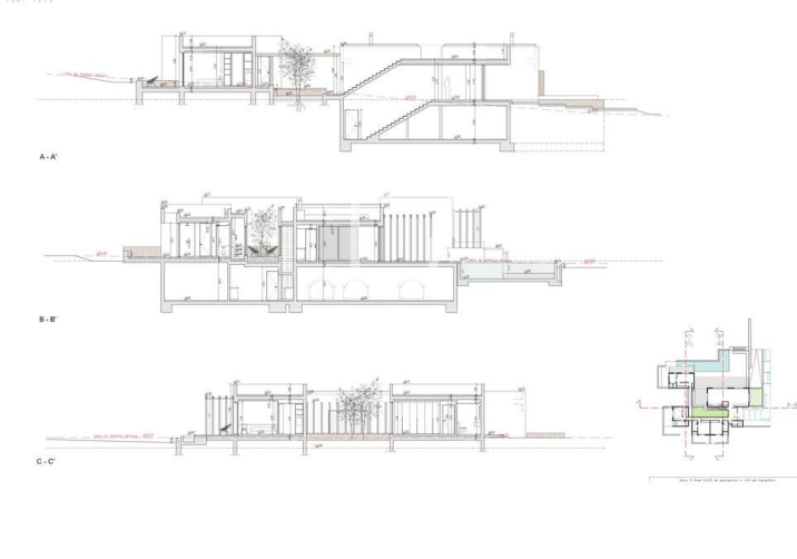
SECCIONES
