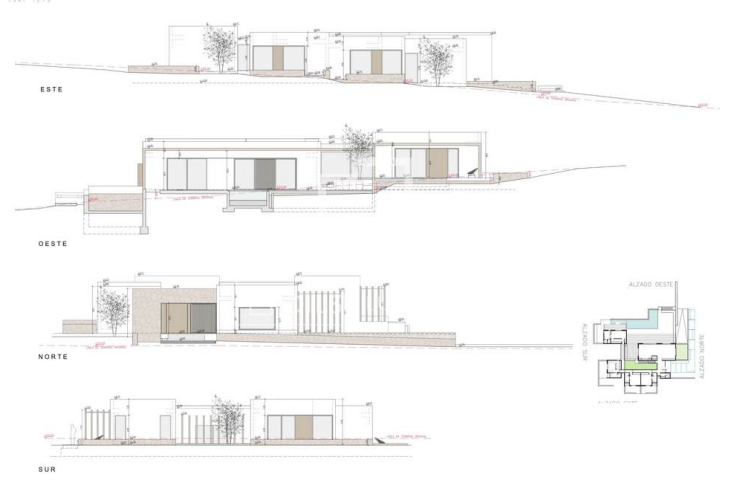
ALZADOS
