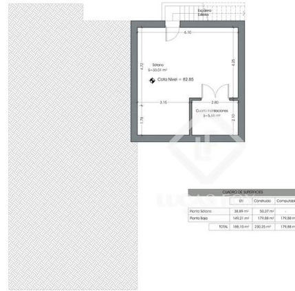
Planta Sótano
