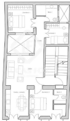
PLANTA PRIMERA
