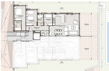
ELS MUNTS RESIDENCIAL PLANO PLANTA BAXA 1A12A
