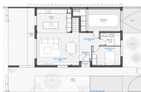
PROJECTE BÀSIC / DISENYOLIG D'UN HABITATGE UNIFAMILIAR APARELLAT AMB PISCINA PLÀNOLS D'ARQUITECTURA A.0
