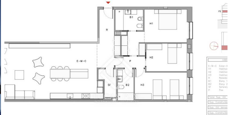
TATGES I LOCAL COMERCIAL "PARCEL·LA 12" AL CLOT D'EMPRIVAT ESCALDES, ANDORRA
