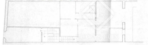
PLANTA PRIMERA
