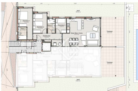
ELS MUNTS RESIDENCIAL PLANO PLANTA BAJA 1A 12A
