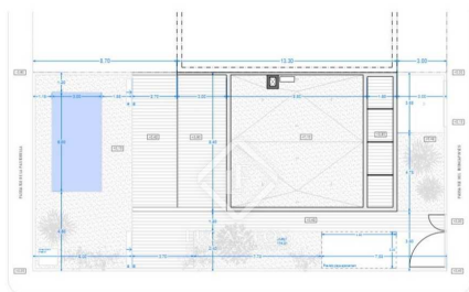
PROJECTE BÀSIC / DISENYOL D'UN HABITATGE UNIFAMILIAR AMB PISCINA PLÀNOLS D'ARQUITECTURA A.01
