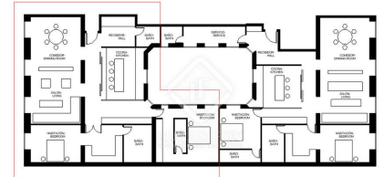
PROPUESTA 2 - PROPOSAL 2 PLANO ARCHITECTÓNICO DE DISEÑO
