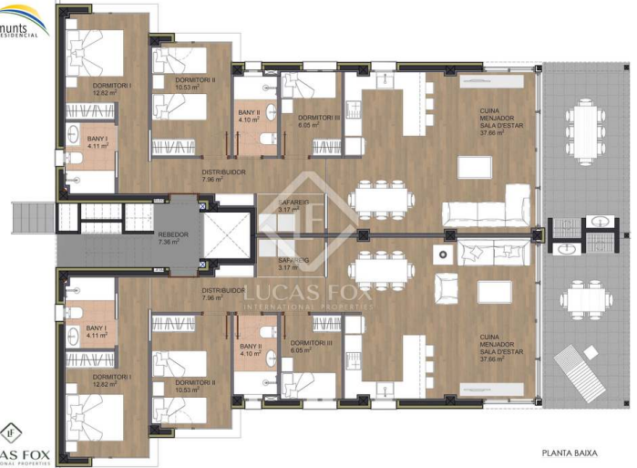
PLANTA BAIXA
