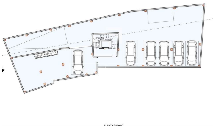
PLANTA SOTANO
