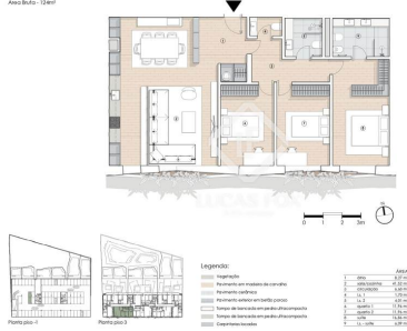
Plano 1 - FRAÇÃO AF - tipologia T3
