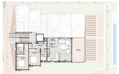
ELS MUNTS RESIDENCIAL PLANO PLANTA PRIMERA 1A 12A
