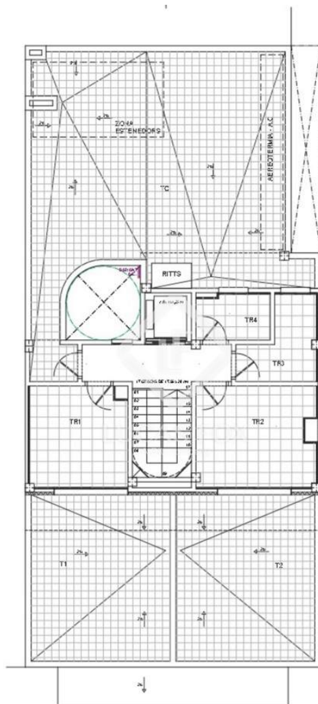
PLANTA SOTACOBERTA E:1/50
