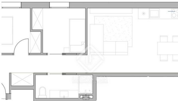
Planta Baixa
