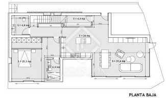
PLANTA BAJA
